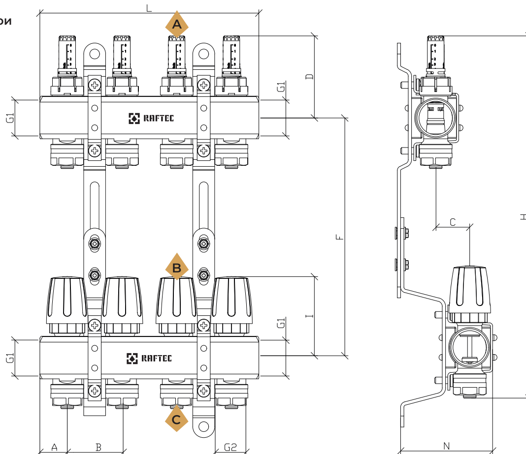
Колекторний блок з витратомірами LCR-1
